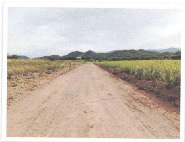
โครงการปรับปรุงซ่อมแซมถนนลูกรังภายในหมู่บ้าน สายบ้านนายอภิรักษ์ หมู่ที่ ๑๗ บ้านทุ่งโป่ง
